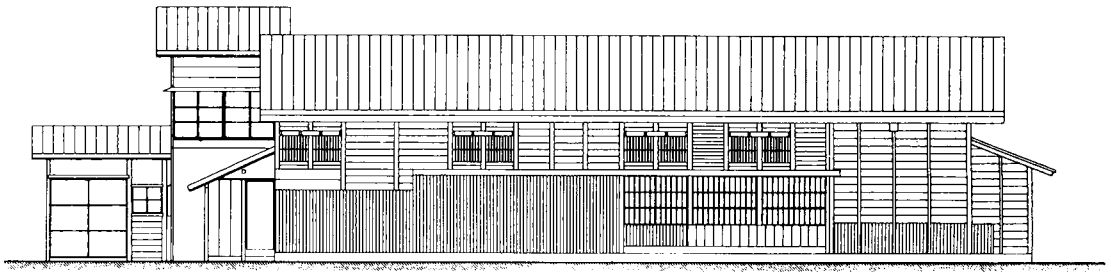
西側立面図
